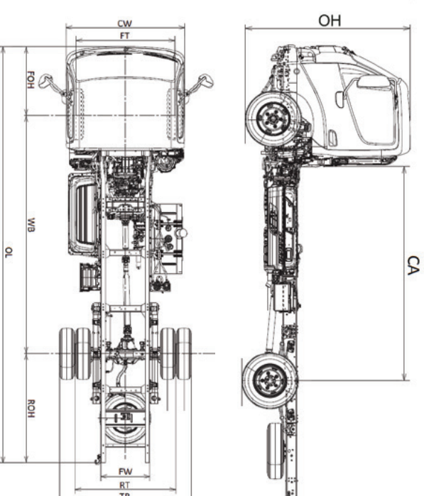
Dimensiones (mm)
